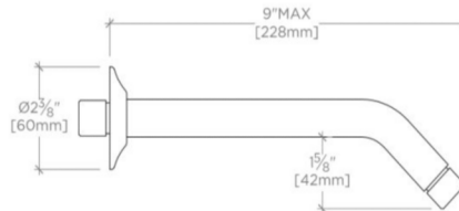
SIDE VIEW SCALE: 3"=1'-0"
