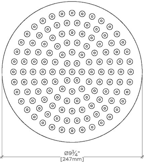
CEILING VIEW SCALE: 3"=1'-0"
