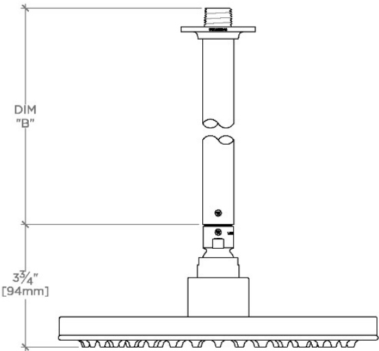
SIDE VIEW SCALE: 3"=1'-0"
