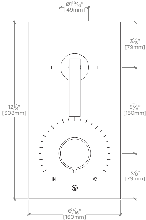
FRONT VIEW SCALE: 3"=1'-0"
