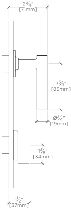
SIDE VIEW SCALE: 3"=1'-0"
