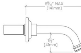
SIDE VIEW SCALE: 3"=1'-0"
