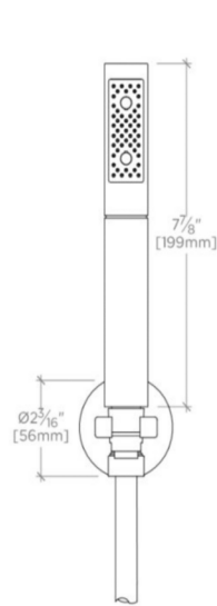
FRONT VIEW SCALE: 3"=1'-0"
