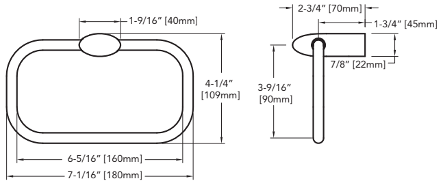
YR416 Towel Ring - Front and Side Views Anillo Para Toalla - Vistas Frontal y Lateral Anneau Porte Serviette - Vue de Face et de Côté
