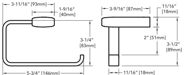
YP630 Paper Holder - Front and Side Views Porta Papel - Vistas Frontal y Lateral Support à Papier - Vue de Face et de Côté
