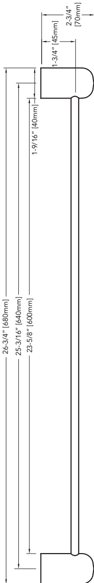
YB416 Towel Bar - Top View Barra Para Toalla - Vista Superior Porte Serviette - Vue de Dessus
