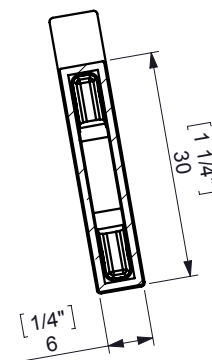
SECCIÓN A-A ESCALA 1 : 1
