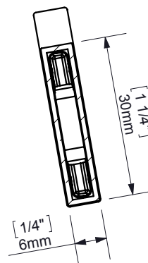
SECCIÓN A-A
