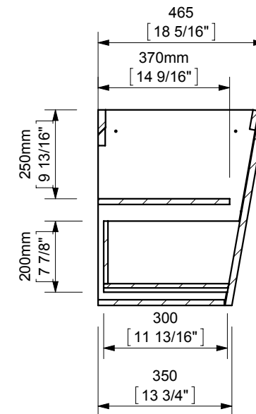
SECCIÓN A-A
