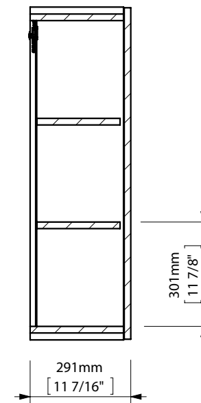
SECCIÓN A-A
