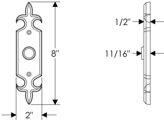
E828 Fleur De Lis Escutcheon 2" x 8"
