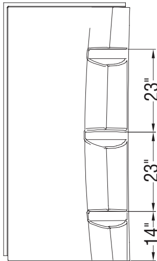
Mur A
