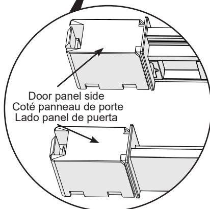
DOOR ON LEFT SIDE CONFIGURATION CONFIGURATION PORTE À GAUCHE CONFIGURACIÓN PUERTA DEL LADO IZQUIERDO
