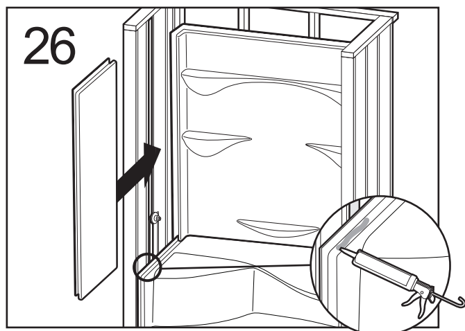
Appliquer du silicone long du rebord intérieur à l'horizontal et à la verticale. Déposer le mur de côté en position.
