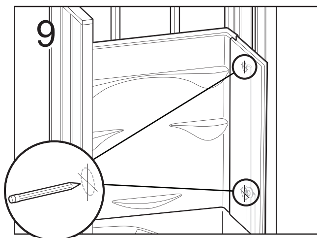
Marquer l'emplacement de la plomberie sur le mur de la douche. Se reporter à la section «Raccord de plomberie installés sur les murs» pour les mesures.
