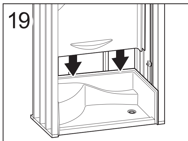
Soulever et placer le mur arrière
