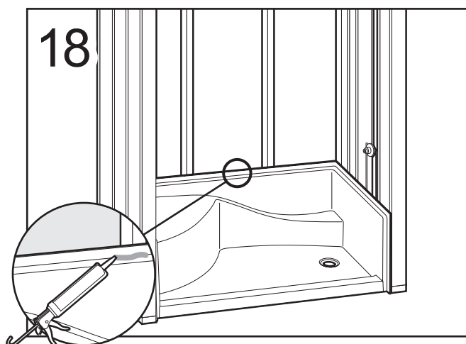
Appliquer du silicone sur le bord horizontal à l'arrière à l'arrière et poursuivre sur une longueur de 8" de chaque côté.
