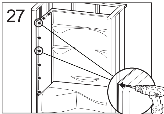
Pré-percer les brides verticales et horizontales devant les montants et les fixer avec des vis.
