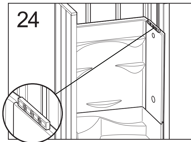
Vérifier le niveau. Ajouter des cales au besoin.
