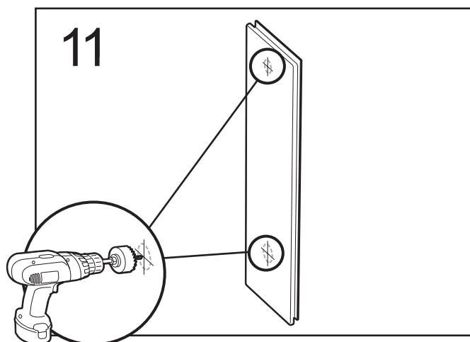
À l'aide d'une scie cloche (denture fine ou tranchant à grain abrasif), faites les ouvertures nécessaires pour le pommeau, la valve et le bec verseur (bain douche), en perçant de l'intérieur (côté lisse) vers l'extérieur.
