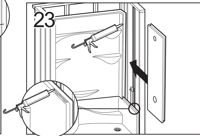
Appliquer du silicone long du rebord intérieur à l'horizontal et à la verticale. Dépoder le mur de côté en position.
