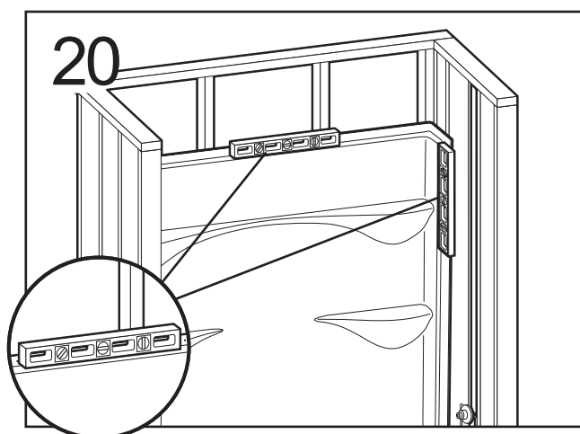
Mettre le mur arrière de niveau horizontalement et verticalement. Utiliser des cales au besoin
