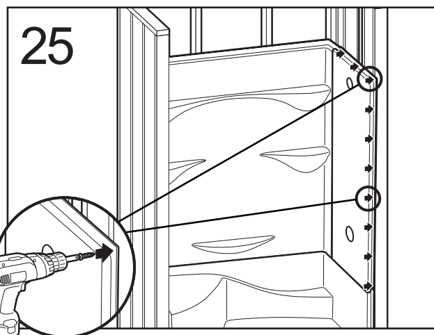
Pré-percer les brides verticales et horizontales devant les montants et les fixer avec des vis.
