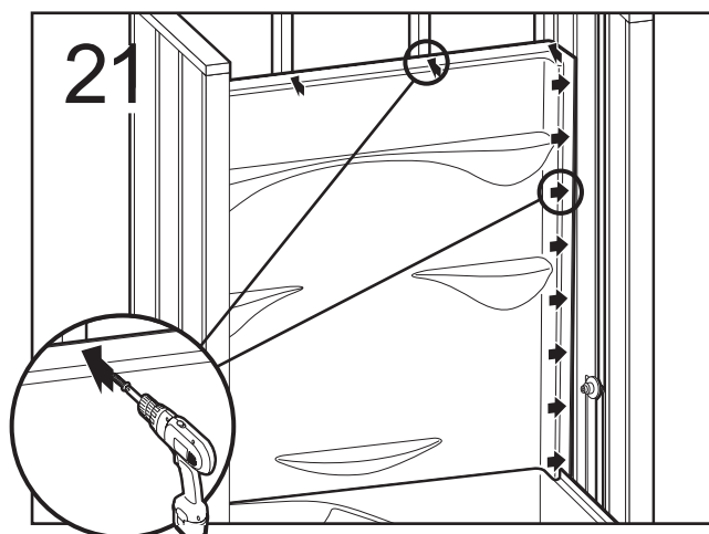
Fixer les brides le long du haut du mur arrière avec des attaches dans chaque montant correspondant. Pré-percer les brides verticales et horizontales devant les montants et les fixer avec des vis.
