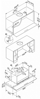
DA 3698, DA 3698 EXT (Installation drawing)
