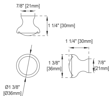
Knob
