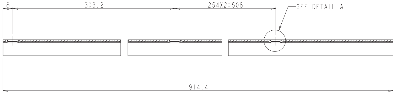
SECTION A-A SCALE 5:8
