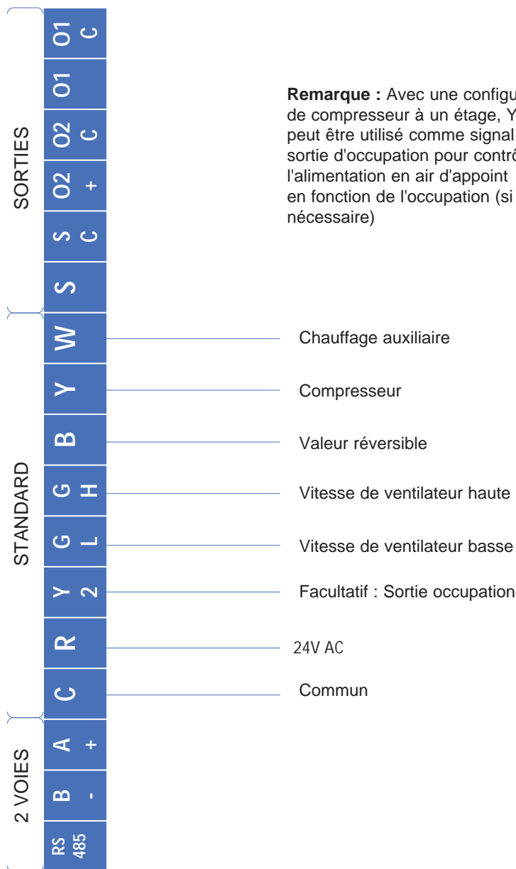
Diagramme 3 : Câblage de communication standard (chaleur : 2 / froid : 1)
