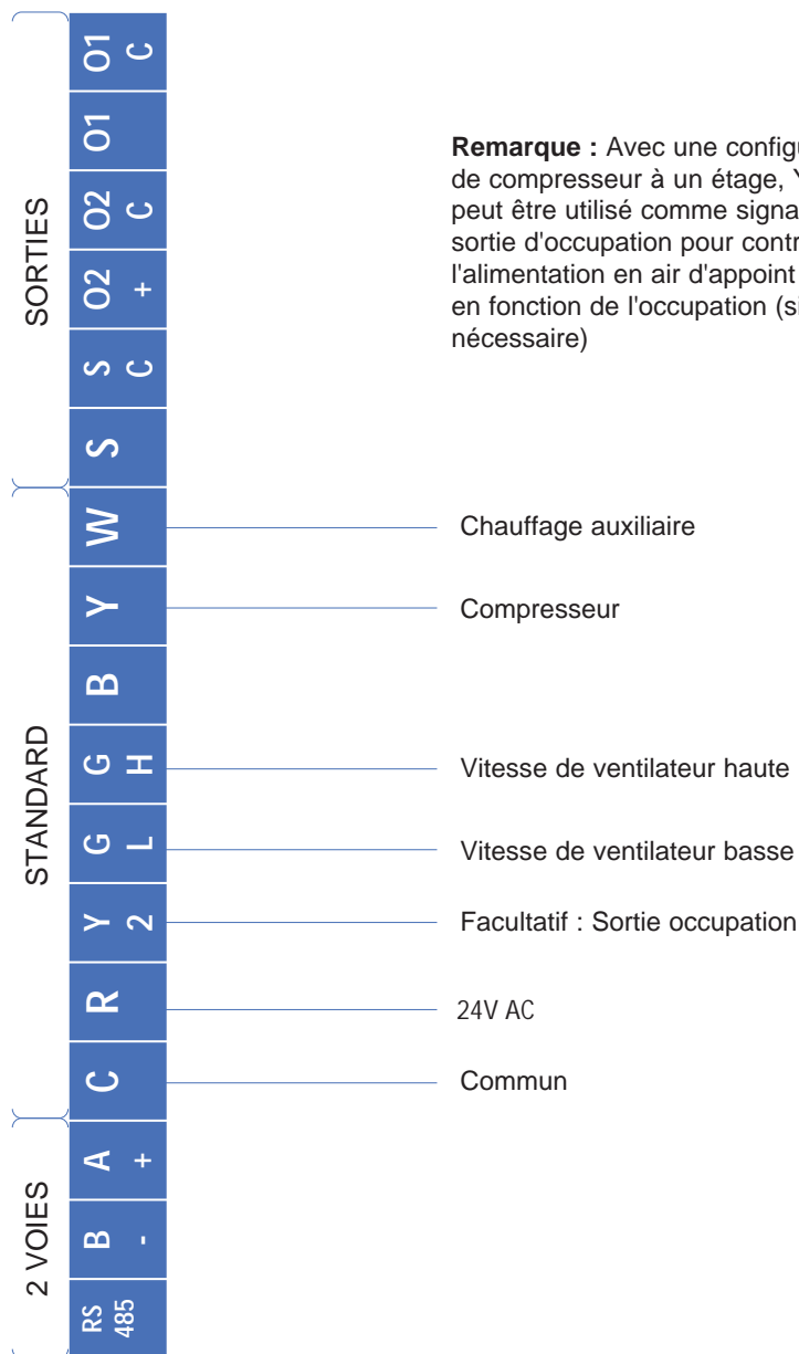
Diagramme 4 : Câblage de communication standard (chaleur : 1 / froid : 1)
