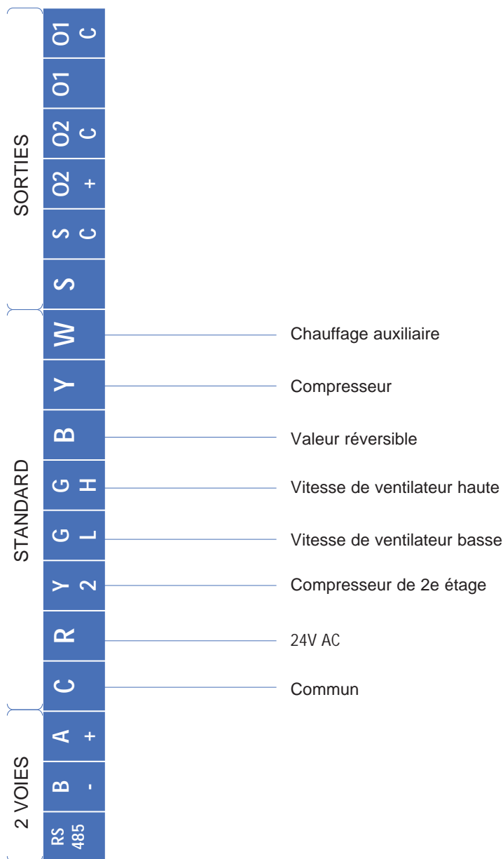
Diagramme 2 : Câblage de communication standard (chaleur : 3 / froid : 2), réglage par défaut en usine
