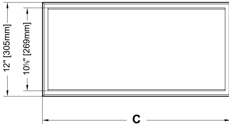
FRONT VIEW VUE DE FACE
