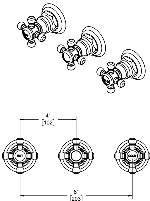
TO-6003L-ZZ shown
