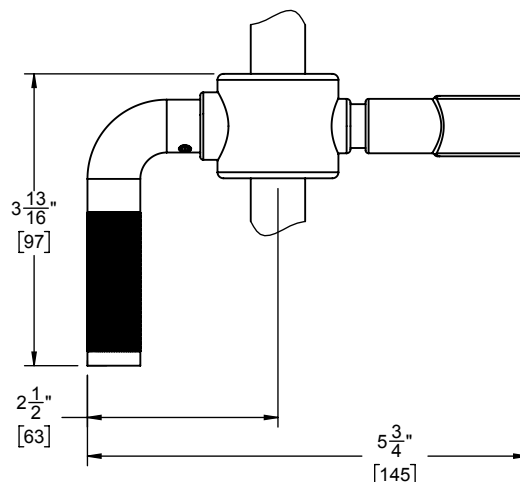
SB-30K/30F HOLDER DIMENSIONS
