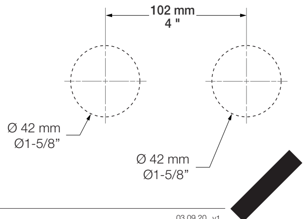
Gabarit de perçage / Hole template
